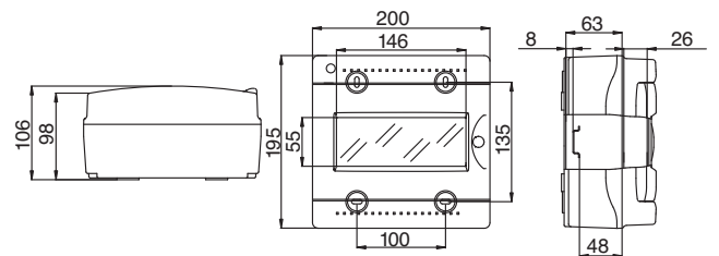
IP65 CE 08 R Codice 05765 IP65 CE 08 GRI Codice 05764
